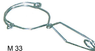
M 33
